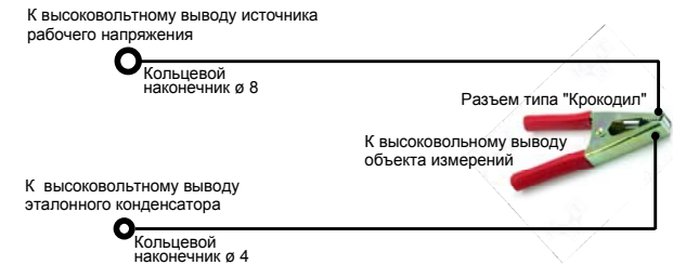
Кабель высоковольтный КВ6 Рисунок 7.8
