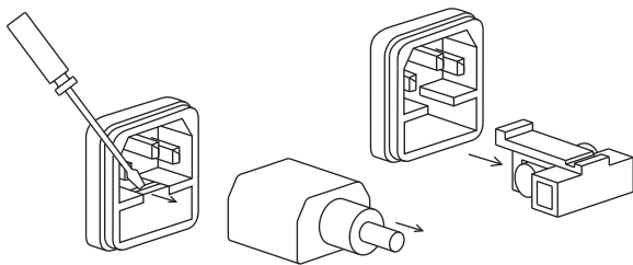
Рис. 31 Замена предохранителя
