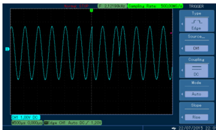
Рис. 66 Осциллограмма сформированного сигнала QPSK
