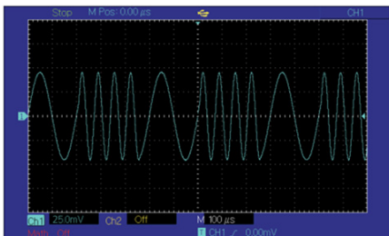
Рис. 35 Осциллограмма сформированного частотно-модулированного сигнала
