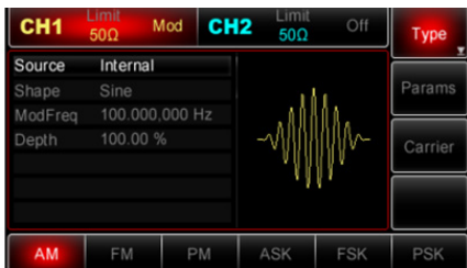
Рис. 22 Выбор источника модулирующего сигнала
