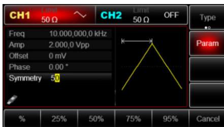
Рис. 14 Установка коэффициента симметрии пилообразного сигнала
