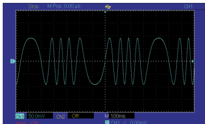
Рис. 42 Осциллограмма сформированного фазо-модулированного сигнала
