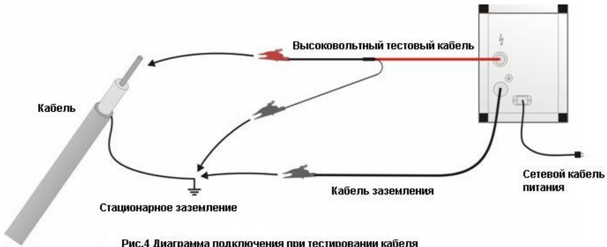
Рис.4 Диаграмма подключения при тестировании кабеля
