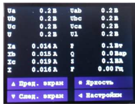
Экран измерений
