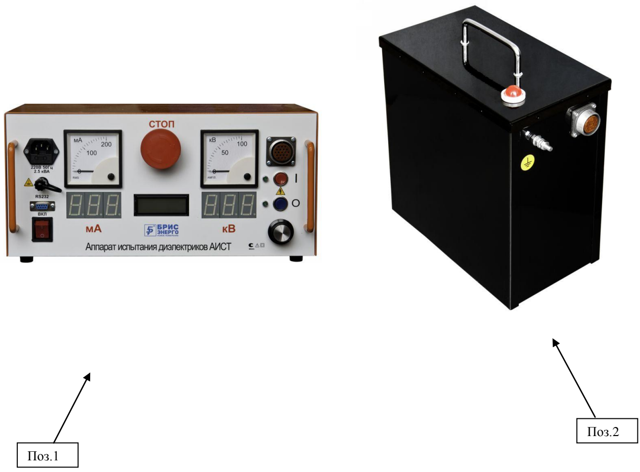
высоковольтный блок (ВВБ) 10кВ – позиция 2 пульт управления (ПУ) - позиция 1 Рисунок 1 Общий вид аппарата
