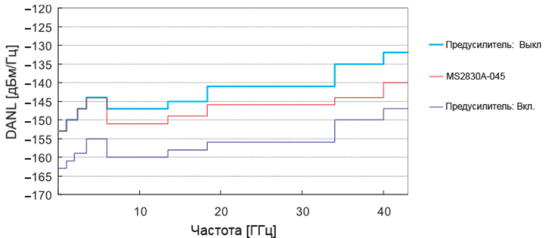
Изменение значения отображаемого среднего уровня шума (DANL) предусилителем (Опц. 068) MS2830A-045 (43 ГГц) С предусилителем, без обхода преселектора
